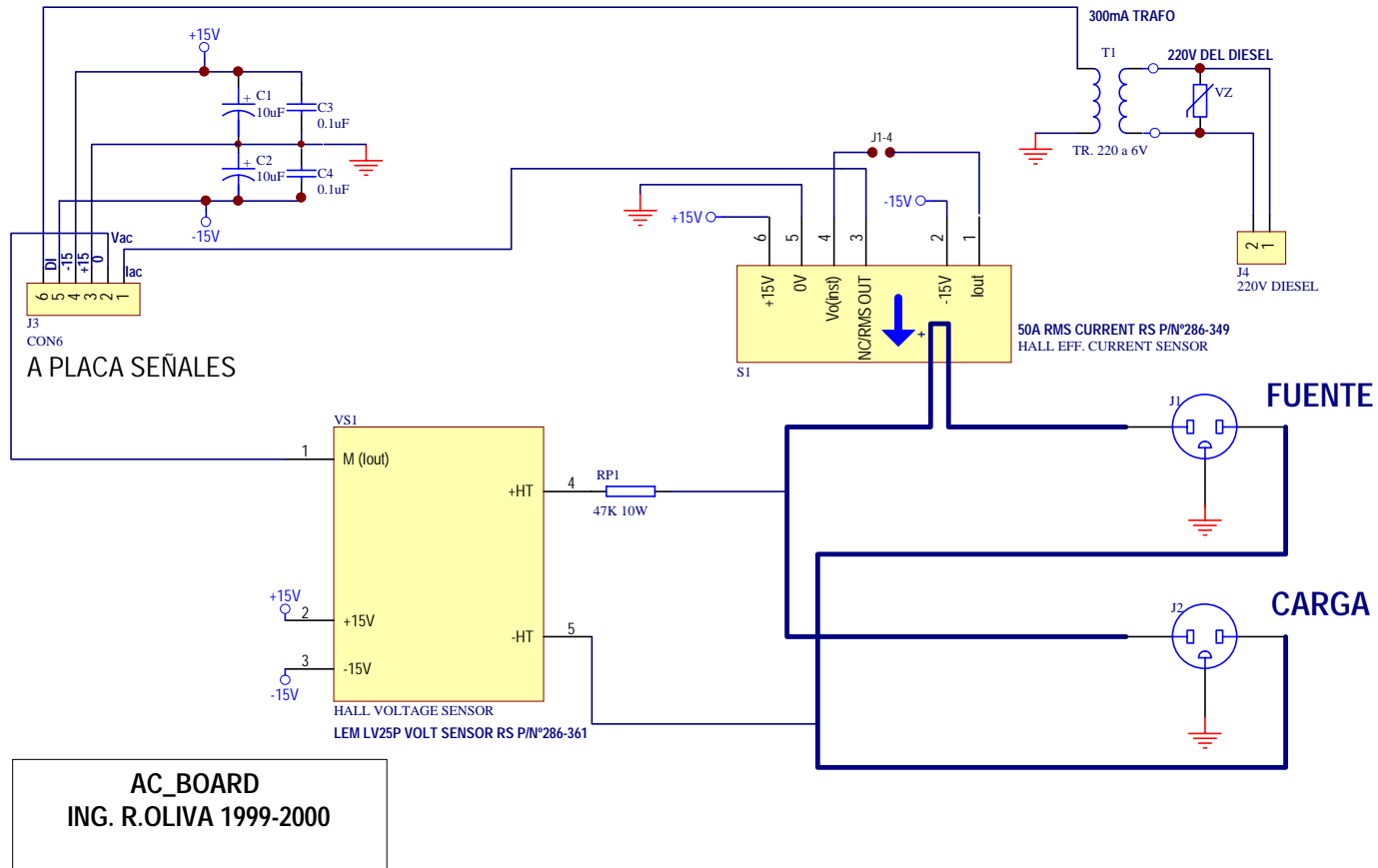
Figura 1: Esquemático AC_BOARD
