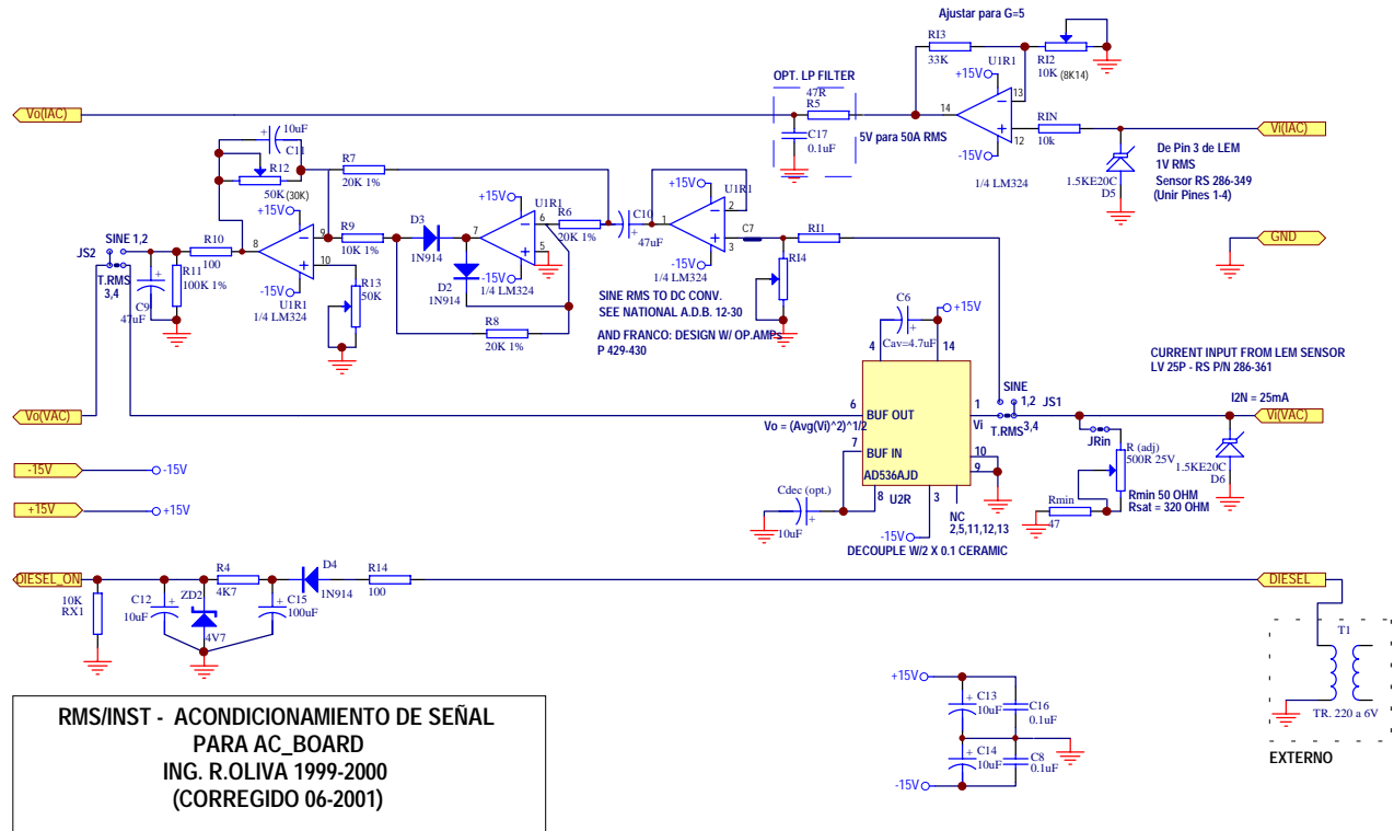
Figura 2 - Esquemático Acondicionamiento de Señal (Típico)
