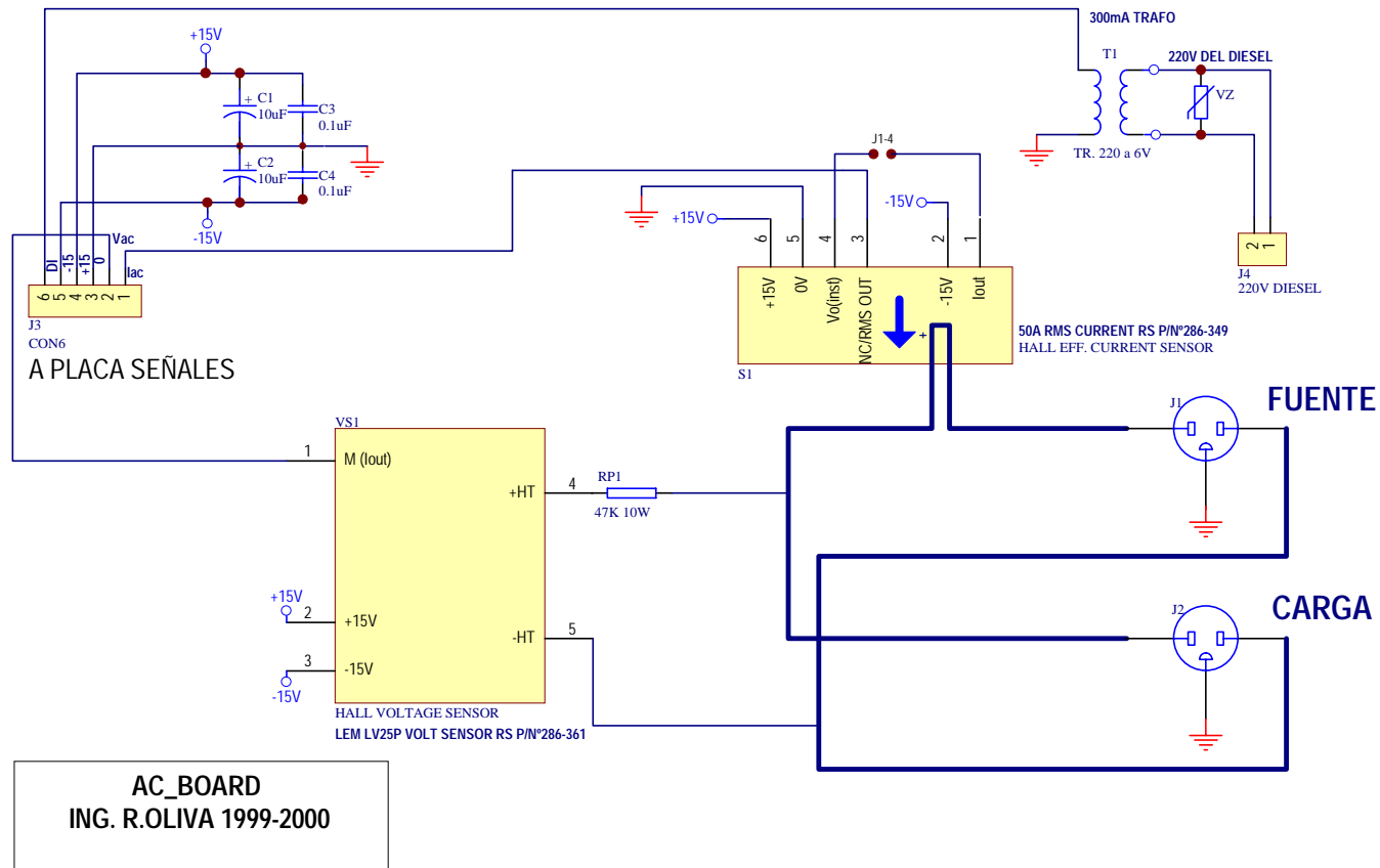
Figura 1: Esquemático AC_BOARD
